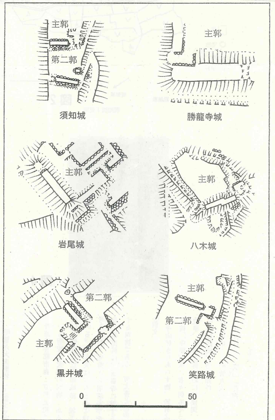
図6 一文字状土塁
