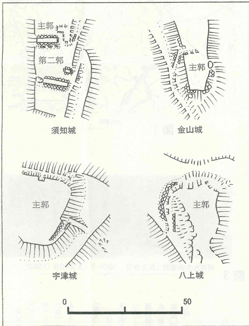
図7 スロープ状の城道
