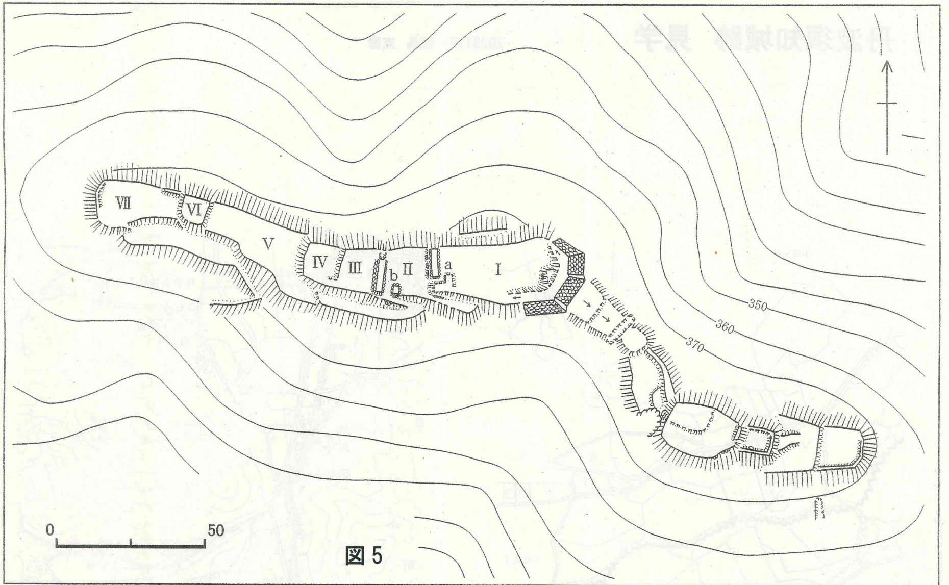
須知城跡縄張り図 (福島克彦調査・作図)
